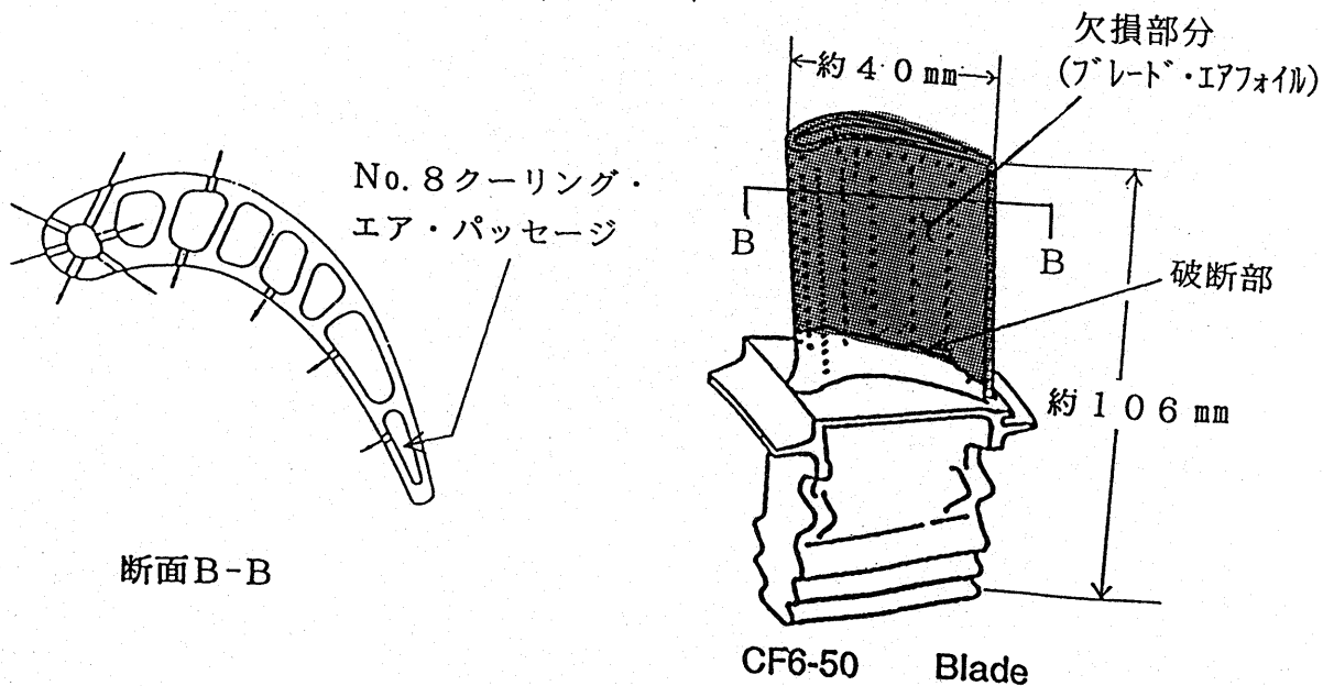
(3) 図B：高圧タービン第1段ブレード
