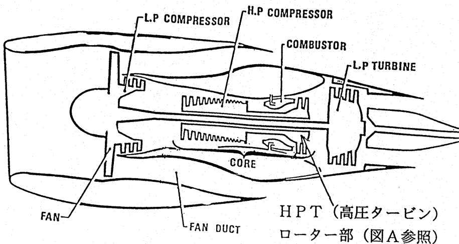
(2) 図A：HPTローター部
