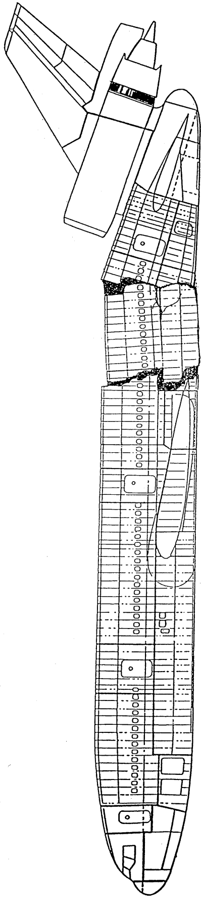
付図3-2 機体の損傷状況図 (左側)
